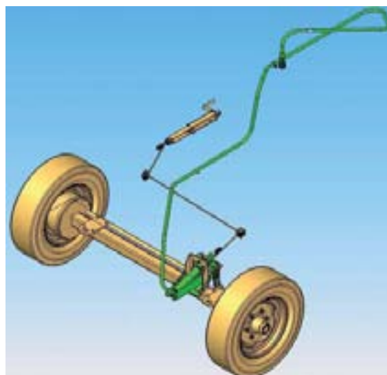
Рис. 7. Гидравлическая тормозная система подметально-уборочной машины ZMC2.0
