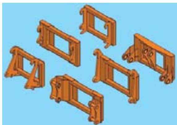
Рис. 5. Системы навески снегоотвалов
