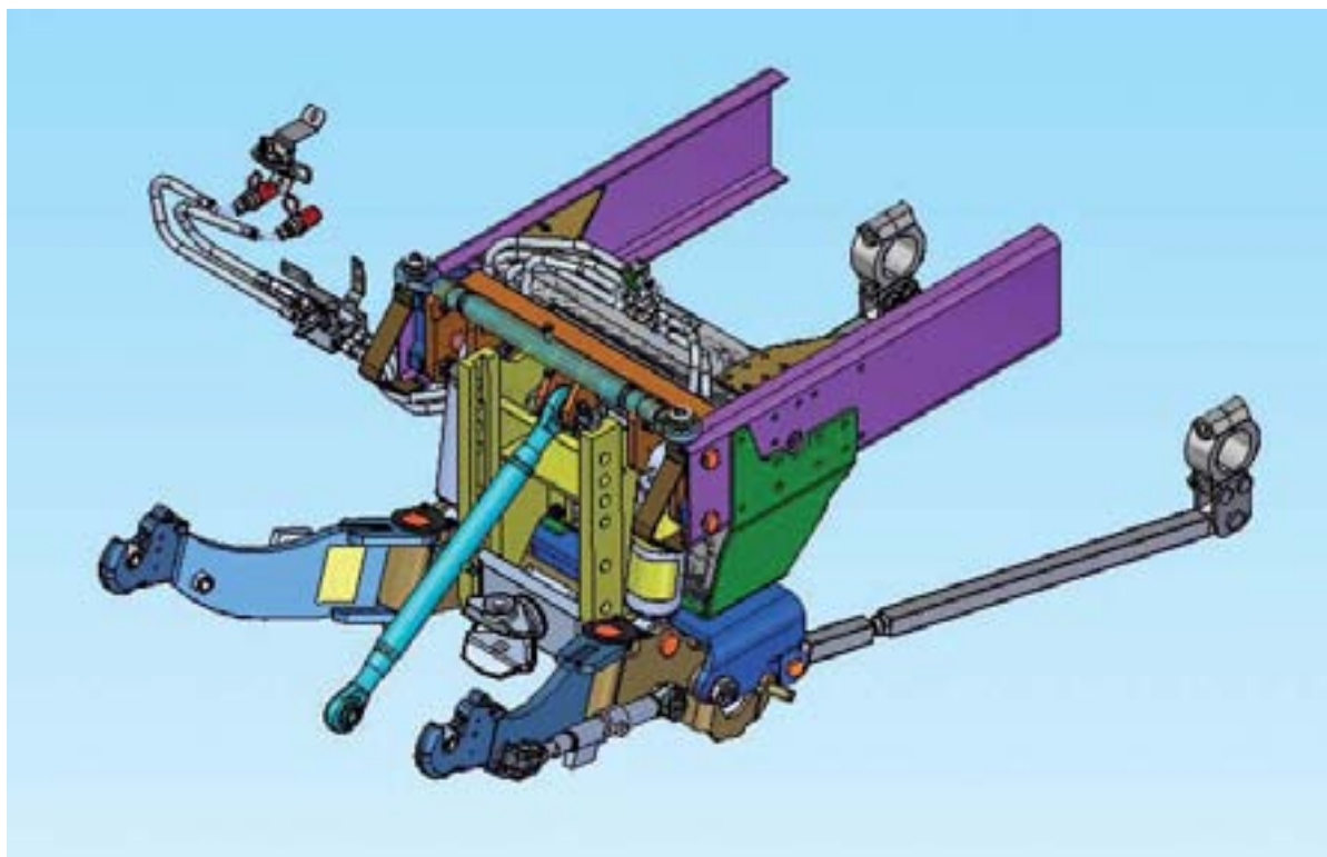
Задняя СТН T-MU4
