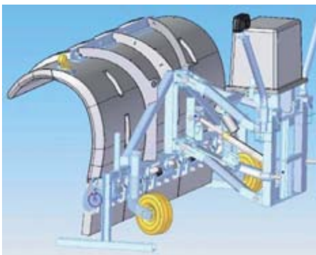
Рис. 1. Снегоотвал с отвалом из ротомолдинга
